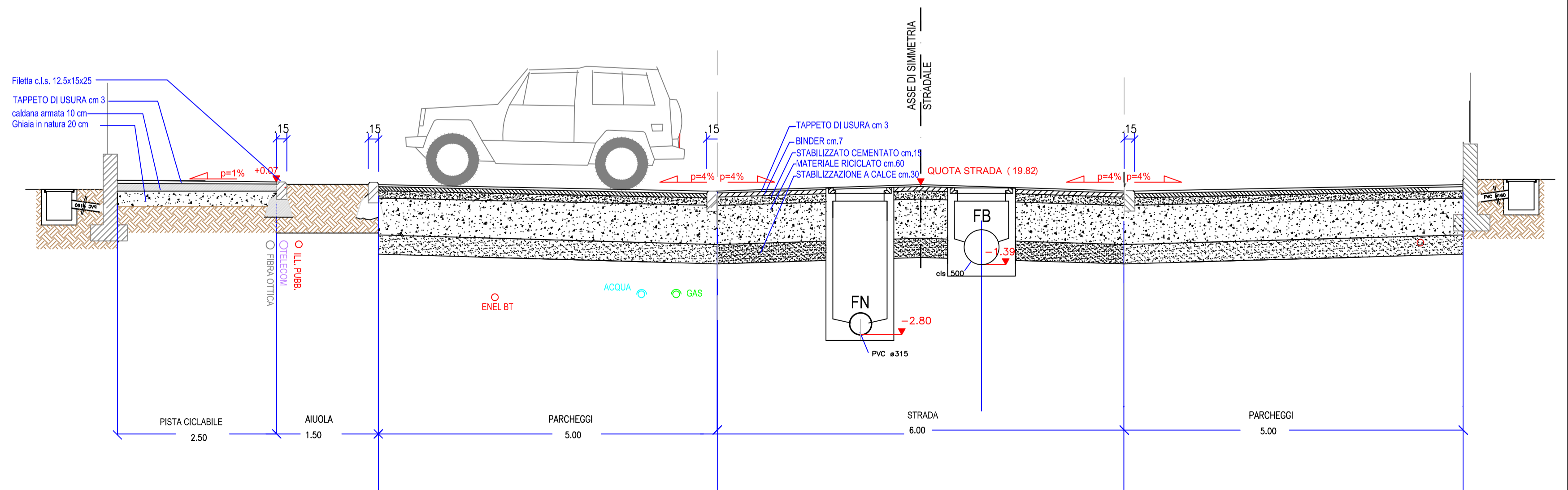
SEZIONE C-C scala 1:50
